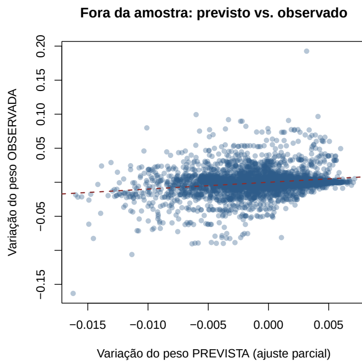
Figura 7: Variação do peso prevista (eixo x) vs. observada (eixo y), fora da amostra. As previsões ficam concentradas perto de zero (o modelo prevê mudanças pequenas), enquanto a variação observada tem bem mais dispersão — coerente com o R^2 baixo da equação (3) (0,038): o modelo capta uma tendência real, mas pequena parte da variação total.
