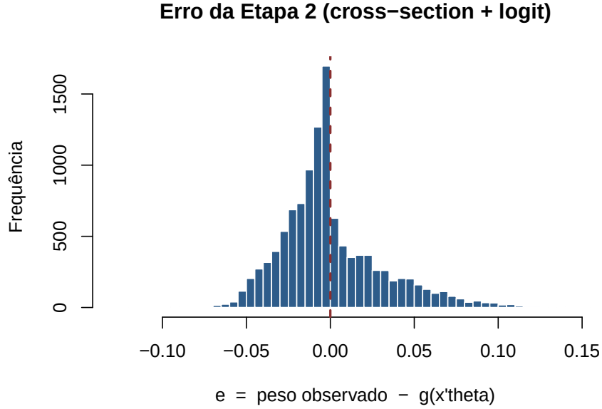
Figura 3: Histograma do erro e da Etapa 2 (11.413 observações). A linha tracejada marca zero.
