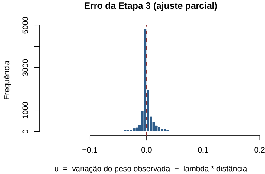
Figura 4: Histograma do erro u da Etapa 3 (10.972 observações). Note o pico estreito perto de zero e as caudas longas — coerente com a curtose alta.
